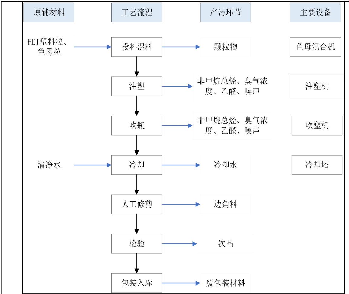
图 2-5 聚酯（PET）容器生产工艺流程及排污节点示意图
