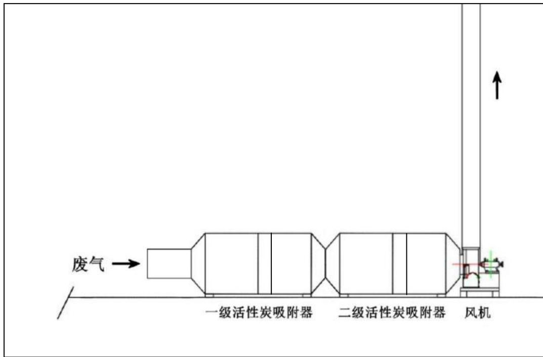
图5.2-1 活性炭吸附装置工作原理示意图
