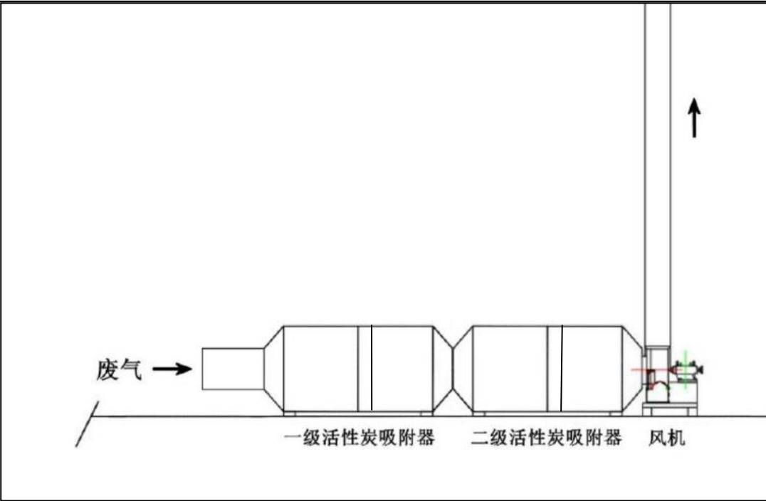
图 4-4 活性炭结构示意图
