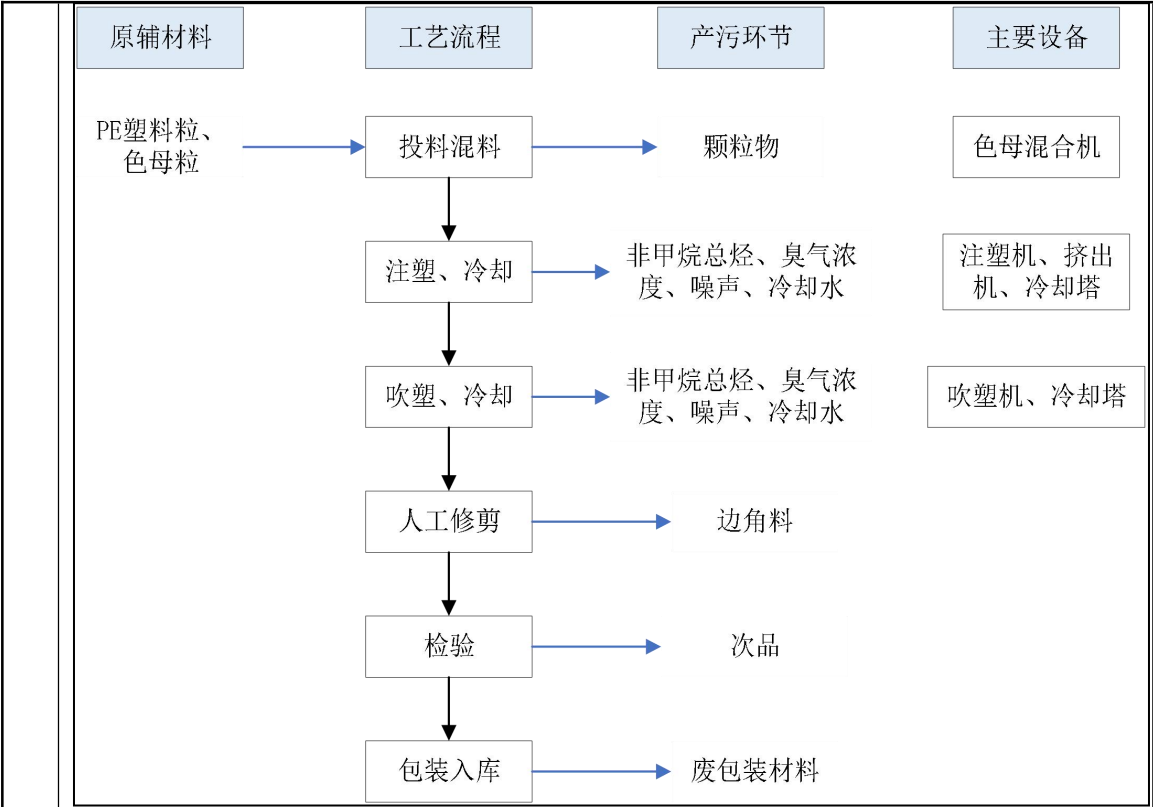
图 2-3 聚乙烯（PE）容器生产工艺流程及排污节点示意图
